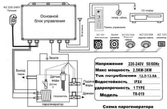
Схема парогенератора
